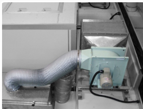
集塵過濾單機/系統運用
