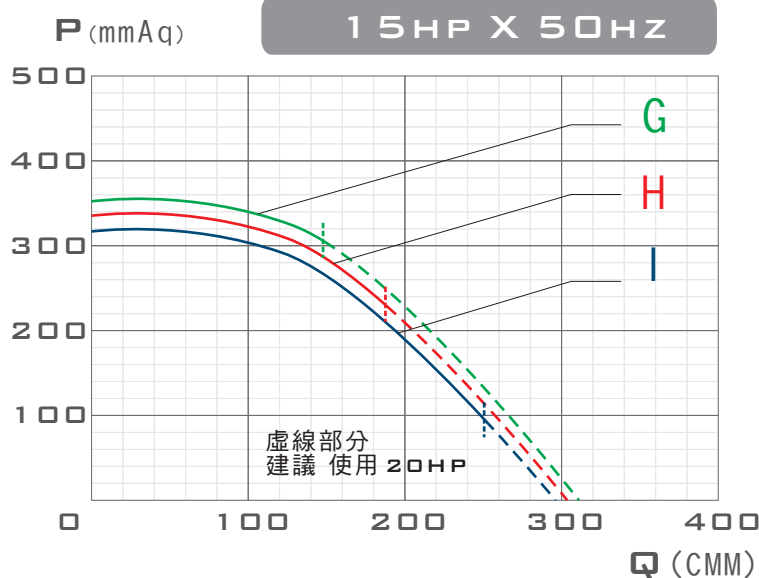
PCH-650 50Hz 性能對照表
