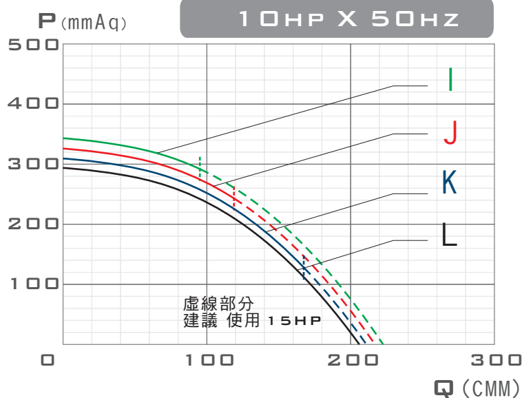
PCH-600 50HZ 性能對照表
