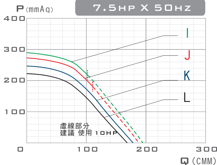
PCH-550 50HZ 性能對照表
