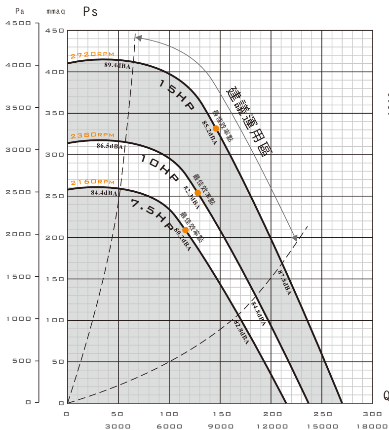
標準性能表 (STANDARD PERFORMANCE DATA)
